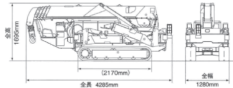
格納状態
