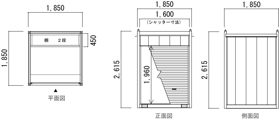
【1 型】 面積／3.42㎡ 約 1 坪 Size／W1,850 × D1,850
