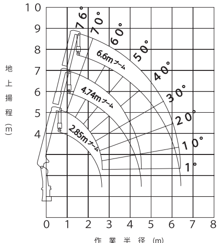
作業半径-揚程図 ※本図はブームのたわみを含んでいません
