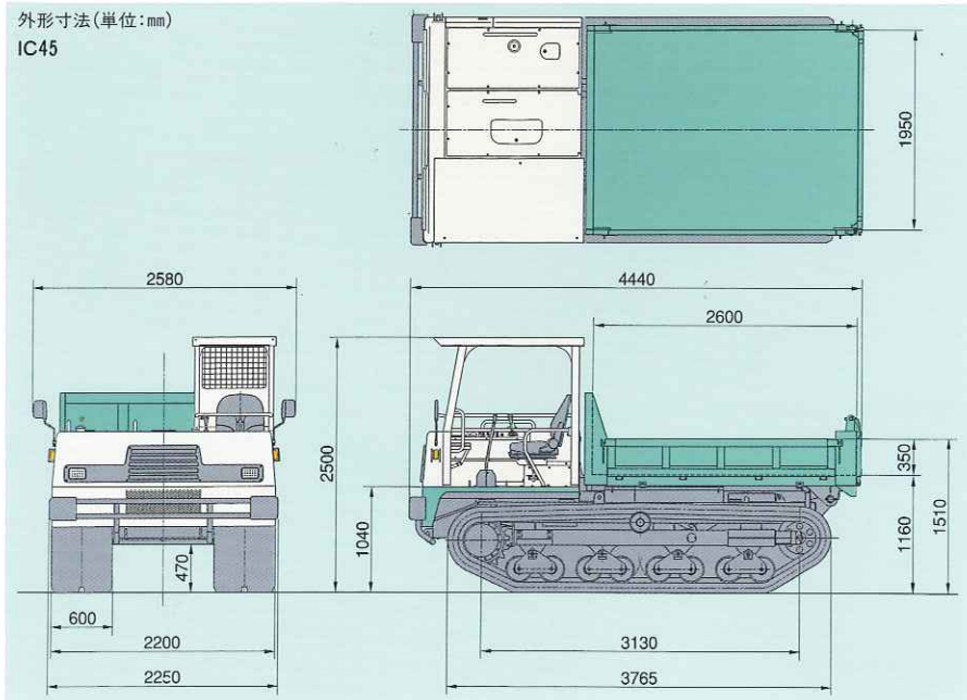
外形寸法(単位:mm)
