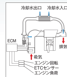
EGRシステム
