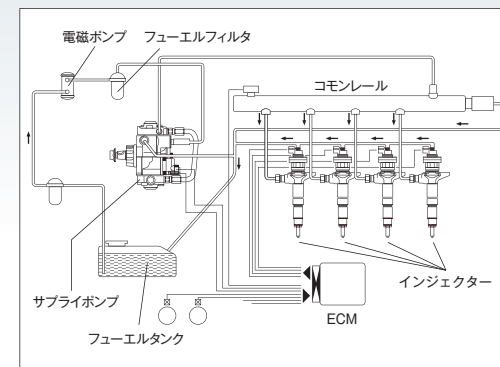
コモンレールシステム(4JJ1)
