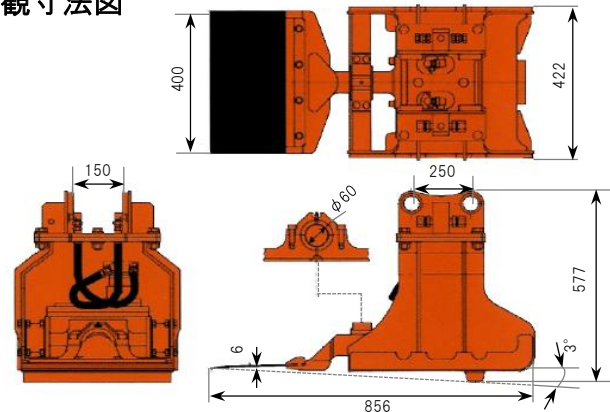
外観寸法図
